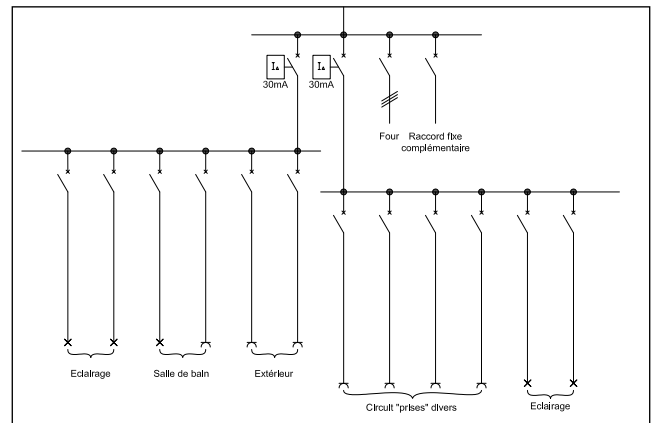
Figure 2: Répartition des circuits sur plusieurs disjoncteurs différentiels de groupe (minimum requis)
