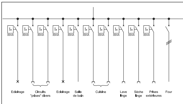
Figure 1: Utilisation de disjoncteurs différentiels / disjoncteurs de ligne combinés (RCD/LS) (Recommandation pour toute nouvelle installation)
