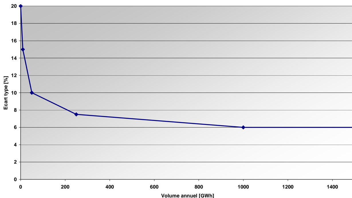
Figure 10: Courbe des écarts types tolérés en fonction du volume énergétique annuel d'un périmètre d'équilibre
