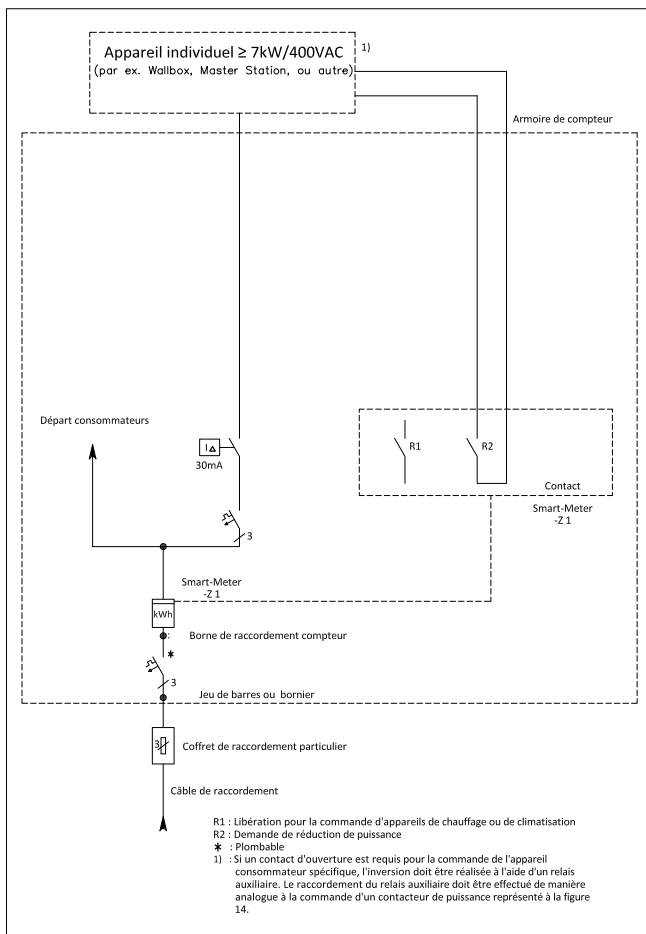
Figure 3: Raccordement d'une borne avec fonction de délestage
